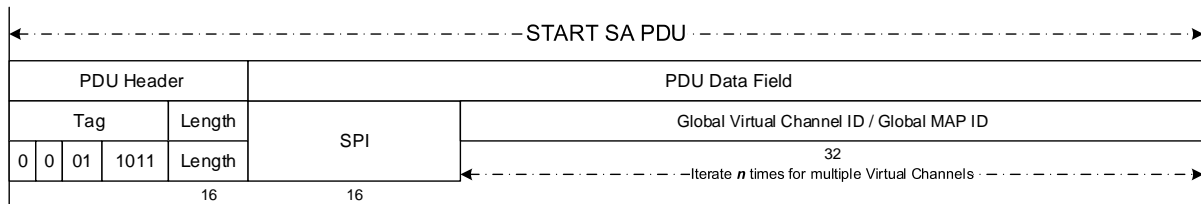
Figure 5-10: Start SA PDU
