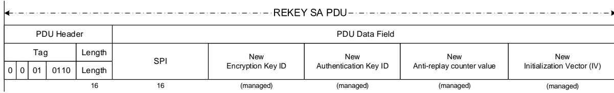
Figure 5-12: Rekey SA PDU
