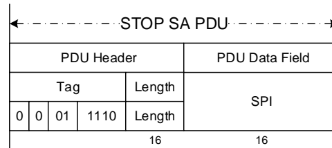
Figure 5-11: Stop SA PDU
