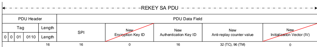
Figure D-8: Rekey SA PDU
