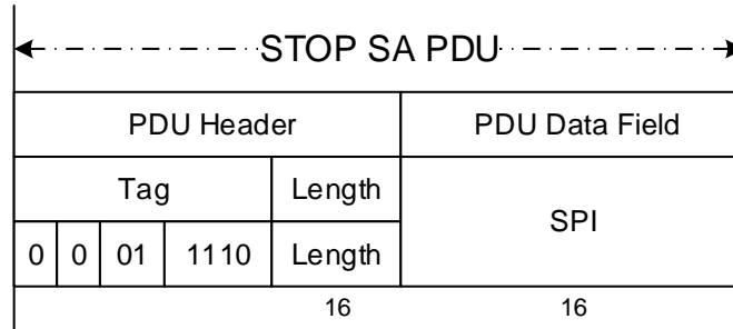
Figure D-7: Stop SA PDU
