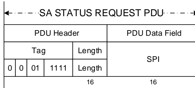
Figure 5-18: SA Status Request PDU
