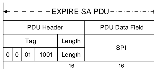
Figure D-9: Expire SA PDU
