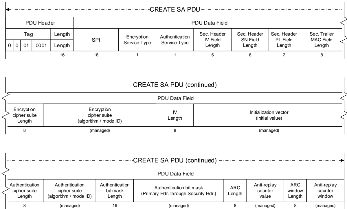
Figure 5-14: Create SA PDU
