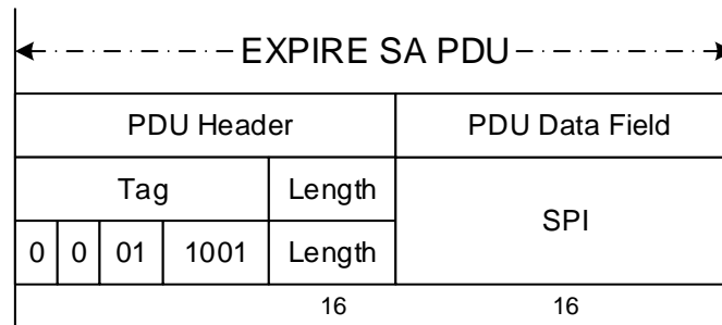
Figure 5-13: Expire SA PDU
